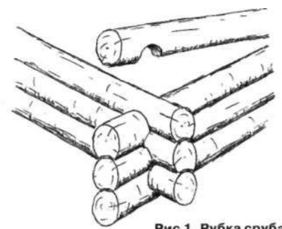
Рис 1. Рубка сруба «в обло»
